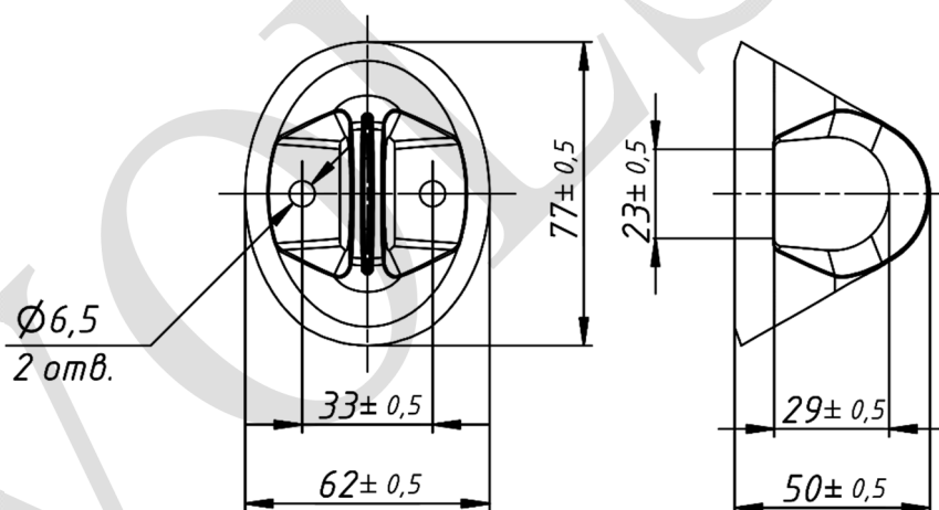
Рисунок 1. Кронштейн VS-РК-01
